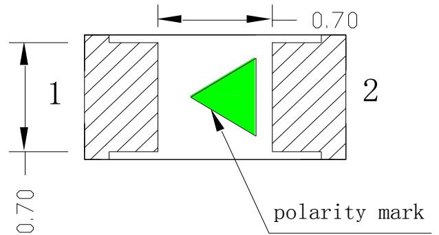
Fig.1-2 Bottom view 背面视图
